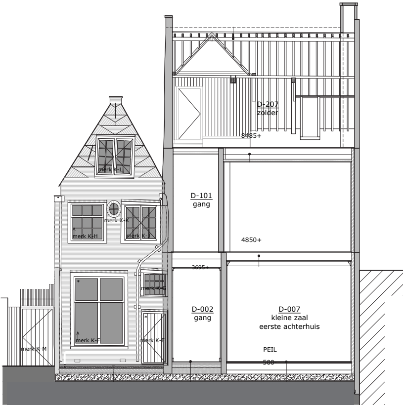
Dwarsdoorsnede
