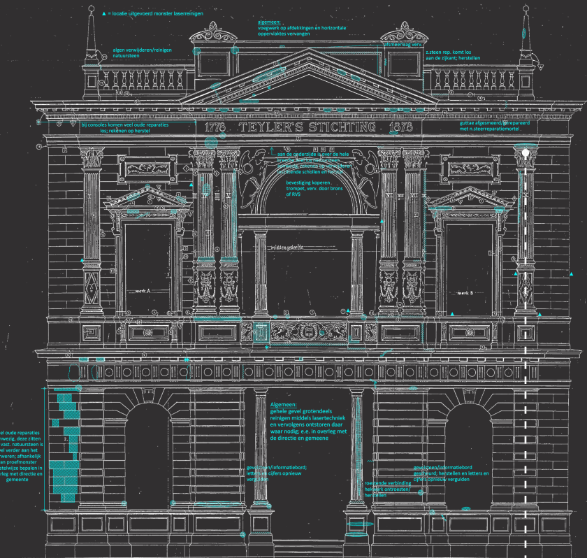
Opname voorgevel
