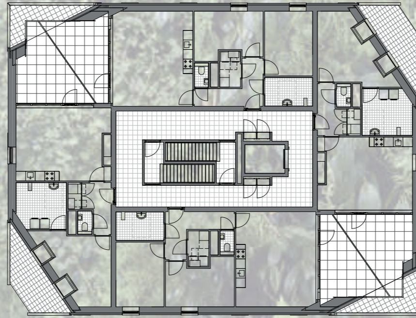
Plattegrond 4e verdieping
