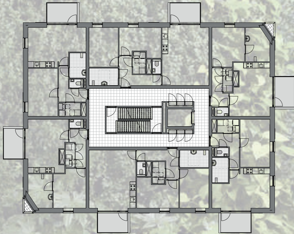
Plattegrond 3e verdieping
