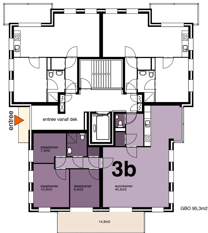
Appartement 3b 95 m² appartement in blok 3
