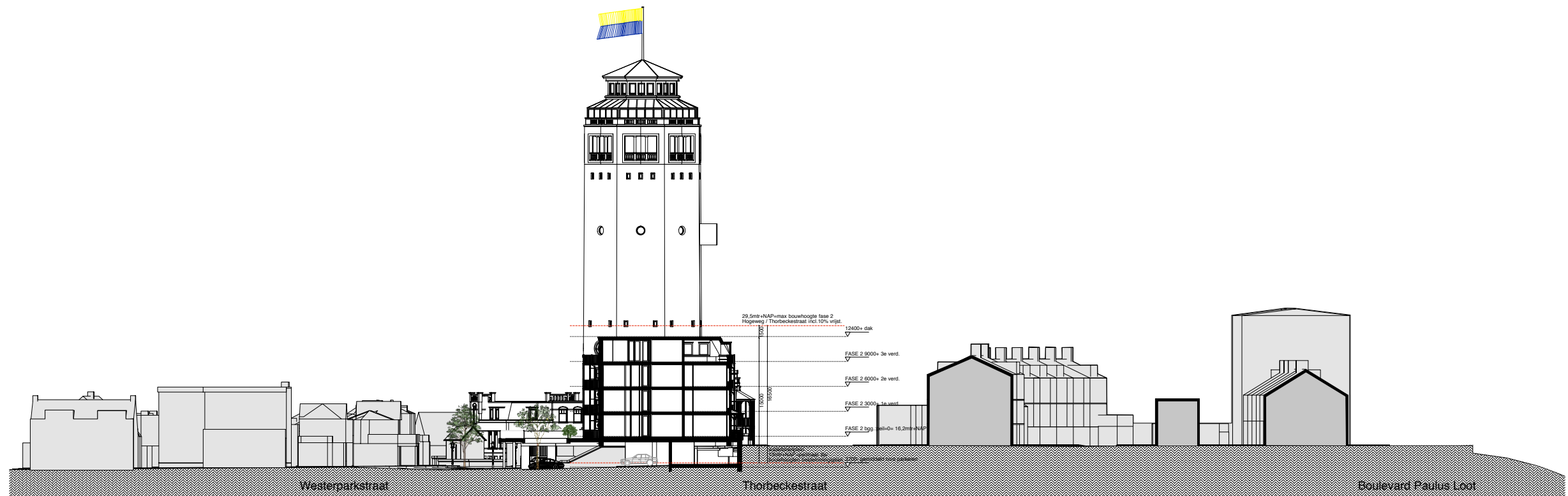
Woonblok doorsnede over blok 4 met de boulevard en het strand aan de rechterzijde
