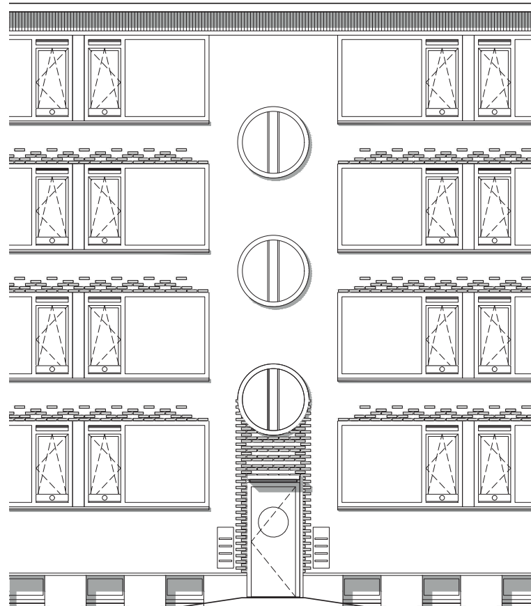
Gevelaanzicht nieuw
