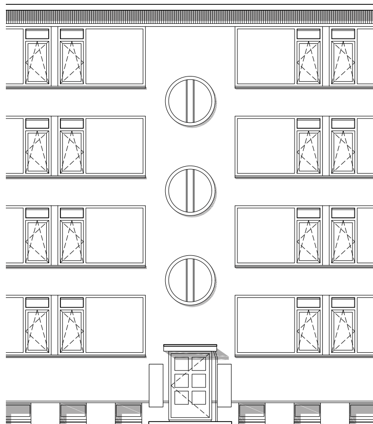
Gevelaanzicht bestaand
