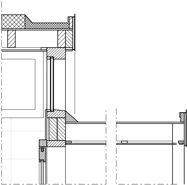
tekening detail stalen boeideel: WVAU Architecten (2021)
