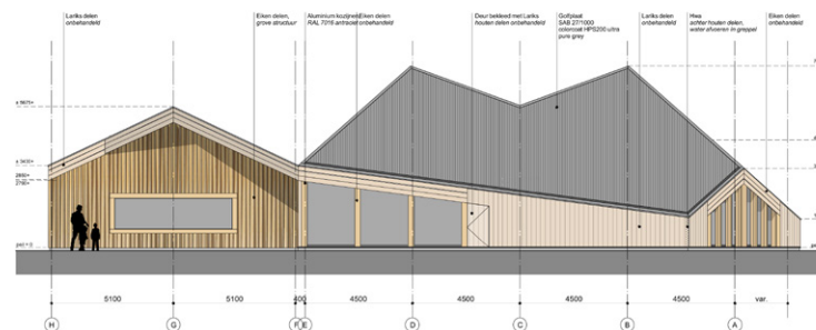
Westgevel
