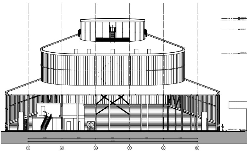
doorsnede AA
