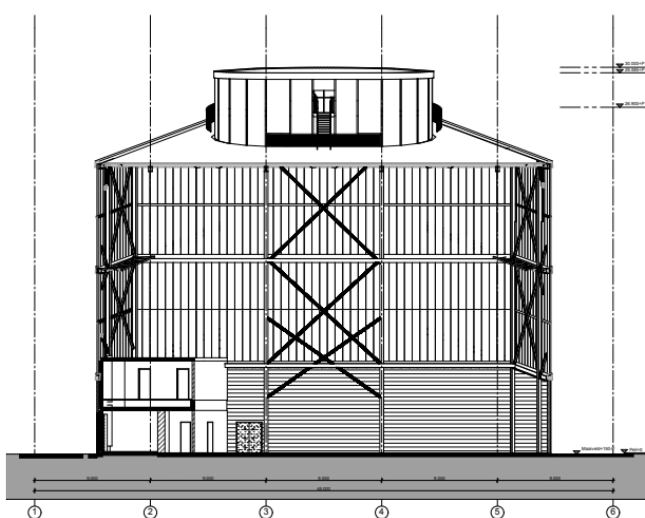
doorsnede CC
