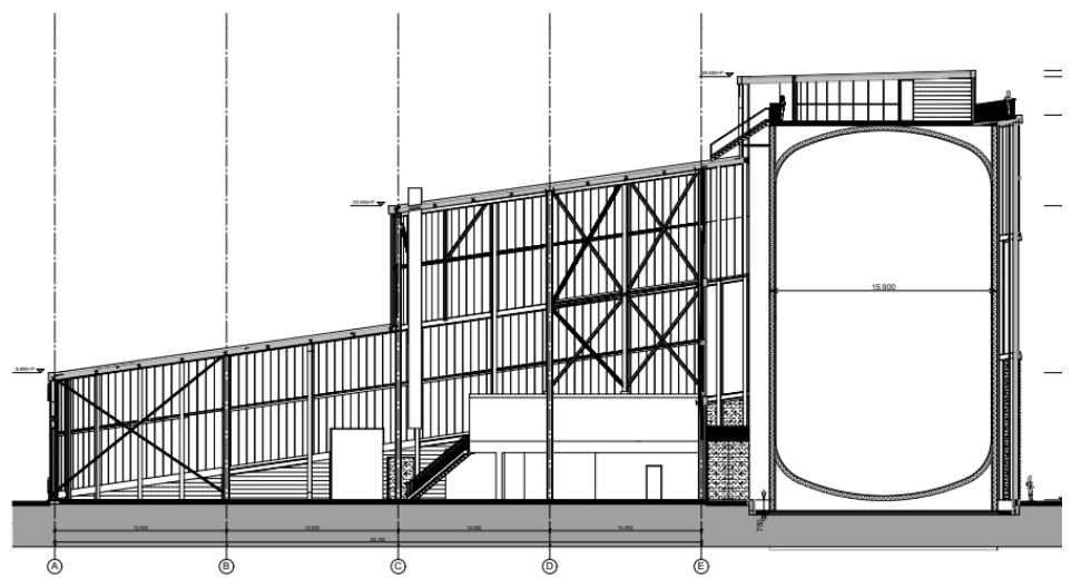
doorsnede BB
