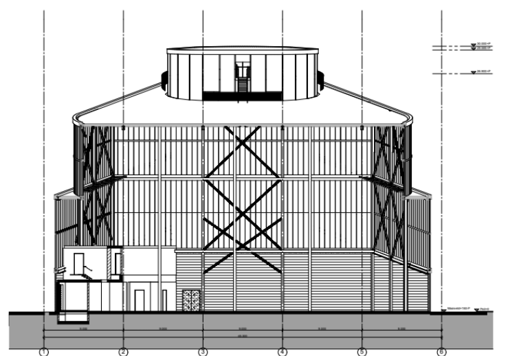
doorsnede DD
