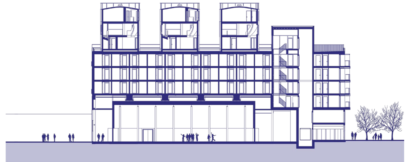
Langsdoorsnede eventruimte
