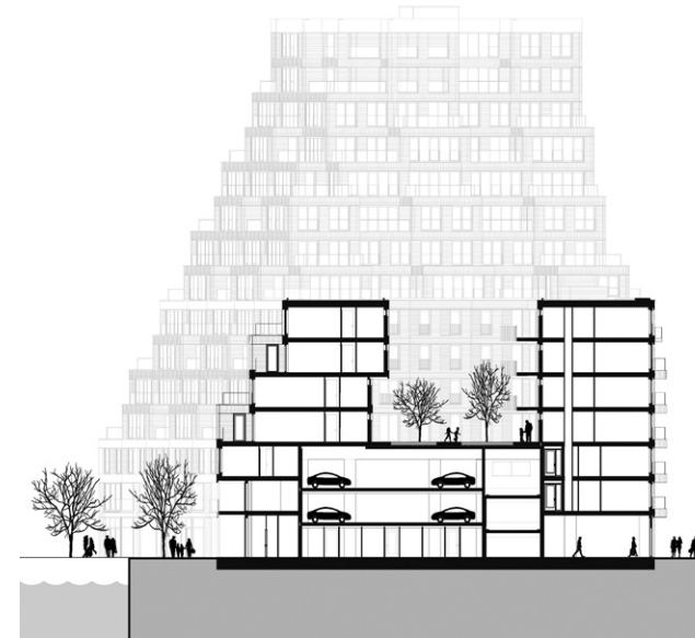
Doorsnede binnentuin
