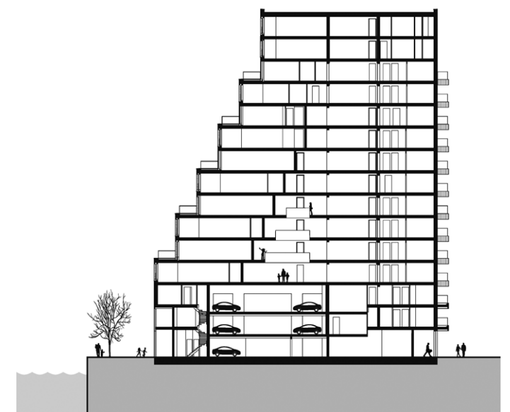
Doorsnede vide in de toren
