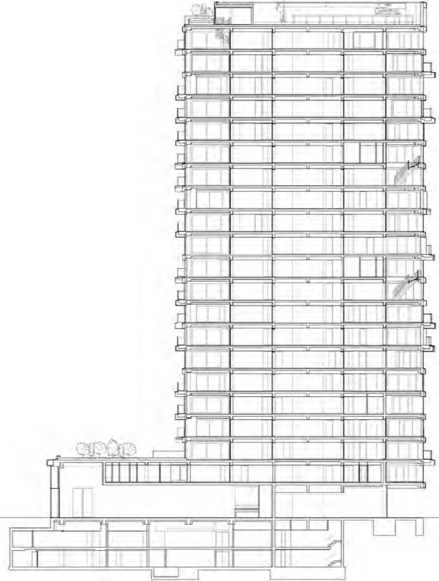
Dwarsdoorsnede
