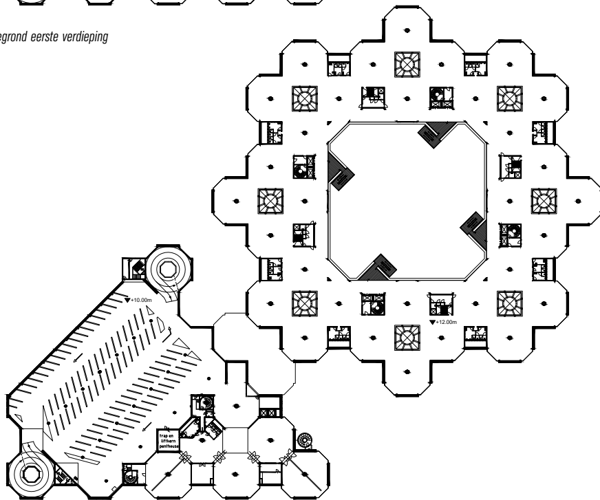
Typische plattegrond
