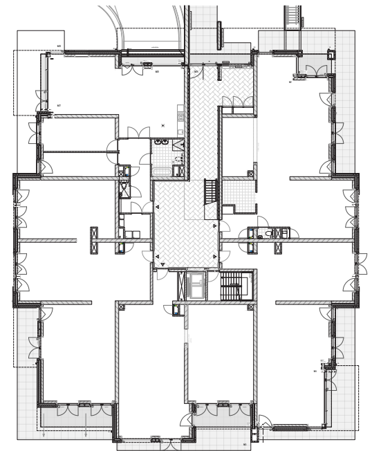
Begane grond
