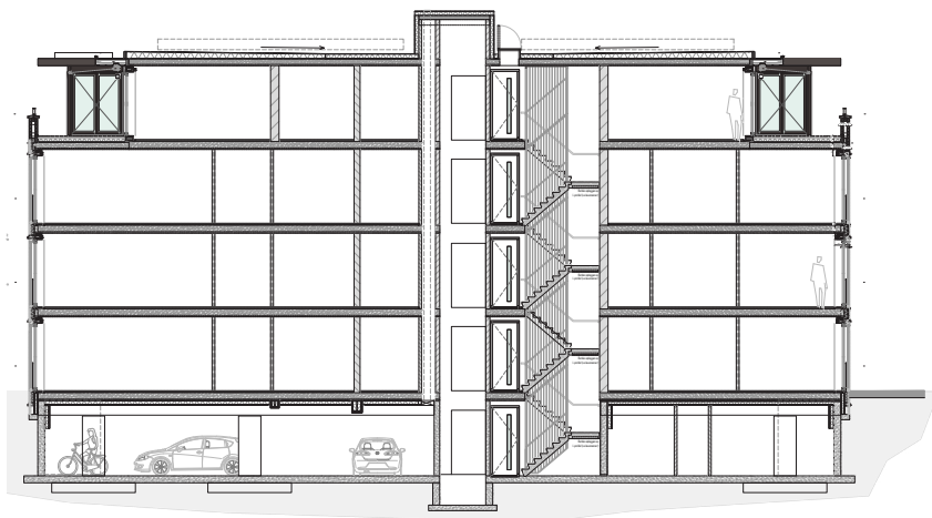
Doorsnede
