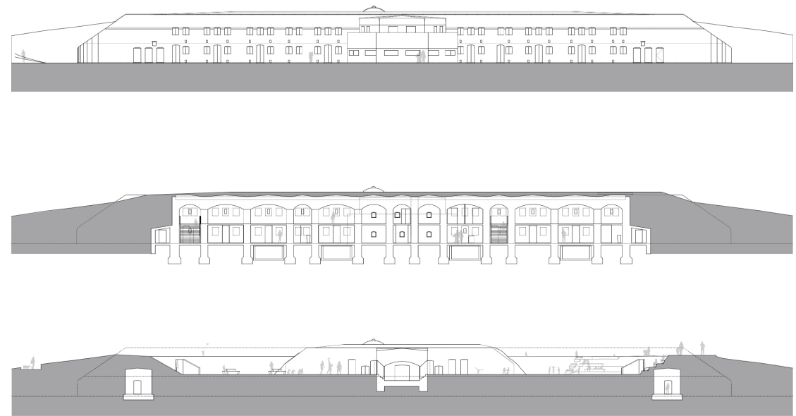
Aanzicht en doorsneden
