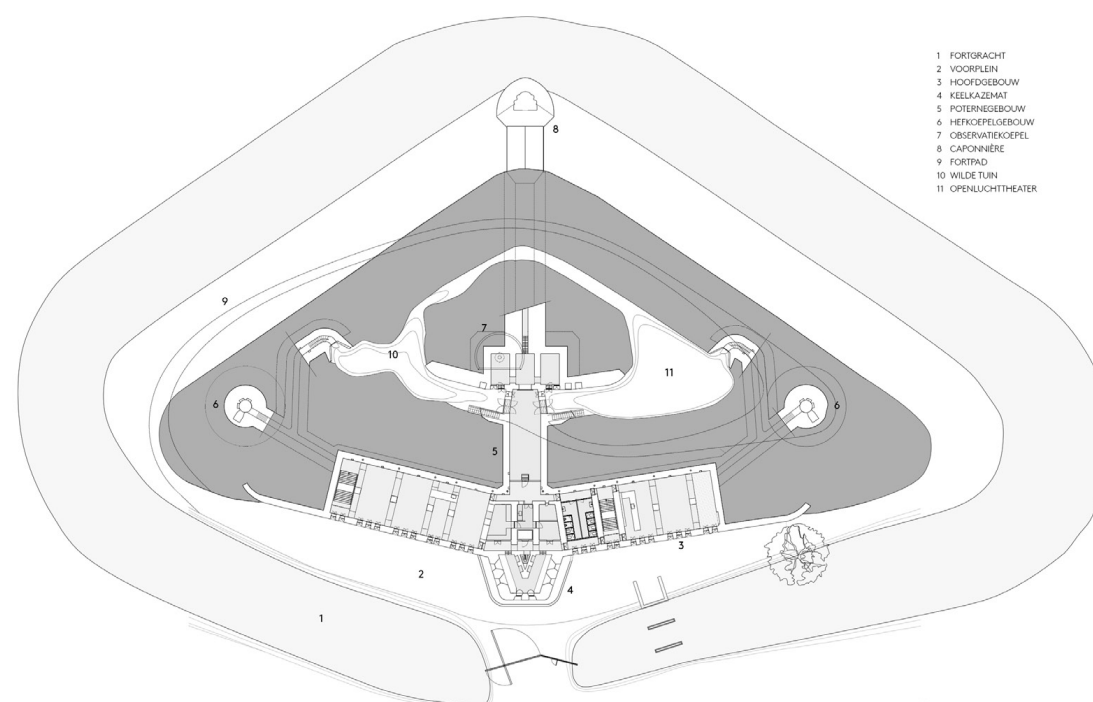
Plattegrond eerste verdieping
