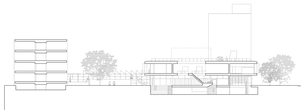
langsdoorsnede over klassieke Rietveld en nieuwbouw
