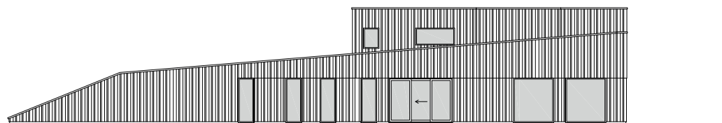
WESTGEVEL
