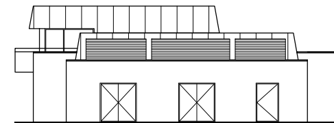
achtergevel zuid
