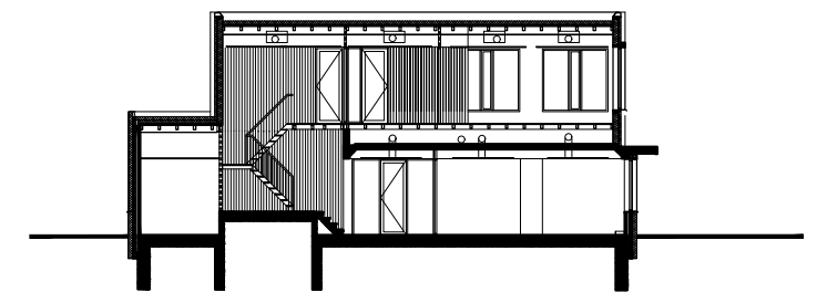
dwarsdoorsnede C-C
