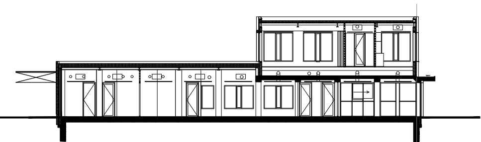
langsdoorsnede D-D
