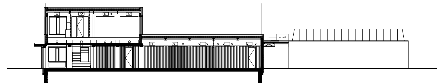
langsdoorsnede B-B
