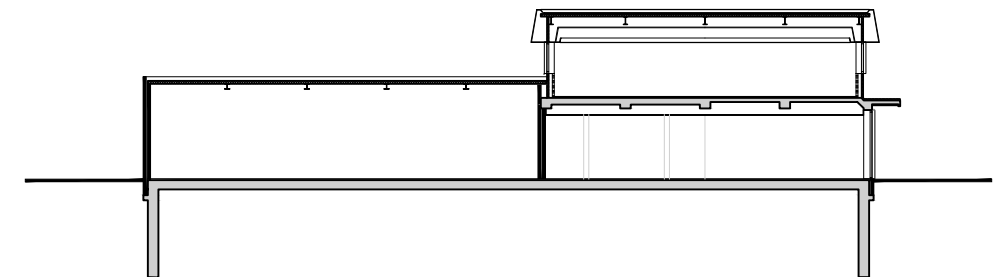
langsdoorsnede A-A
