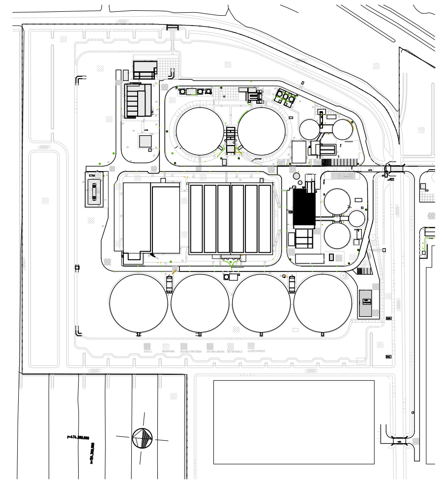
situatie
