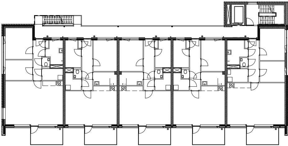
plattegrond 2° verdieping
