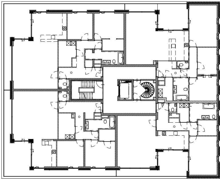
plattegrond 1° verdieping
