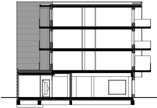
principeddoorsnede
