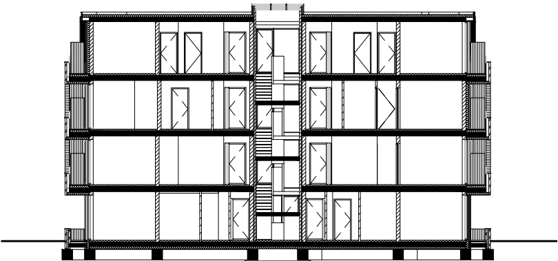
principeddoorsnede
