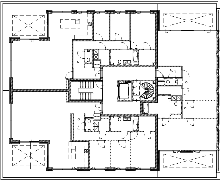
plattegrond 3° verdieping
