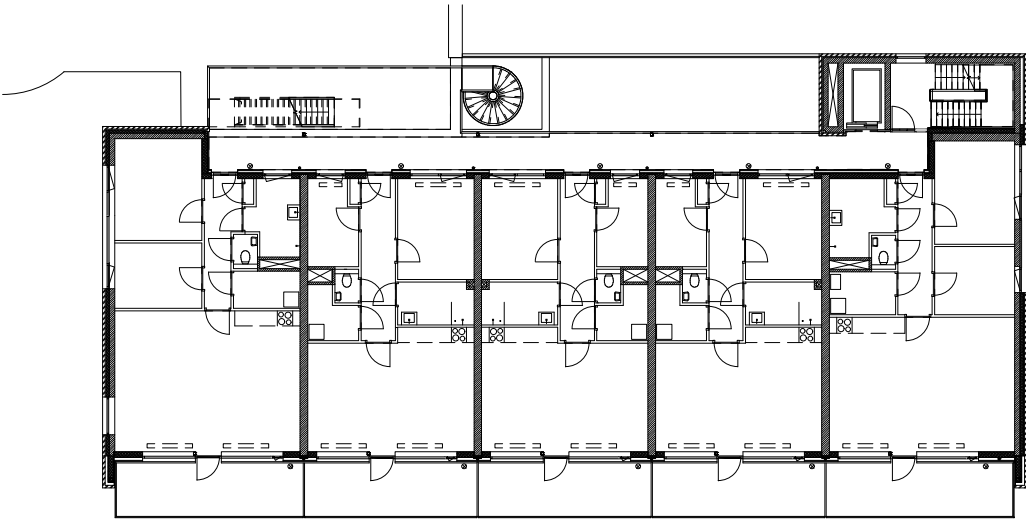
plattegrond 1° verdieping
