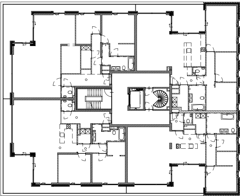
plattegrond 2° verdieping
