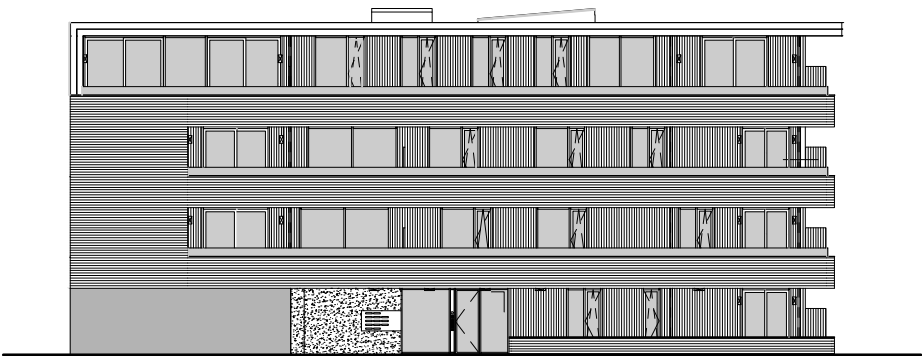
westgevel
