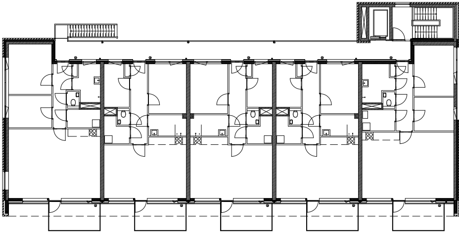
plattegrond 3° verdieping
