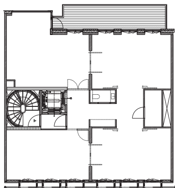
tweede verdieping
