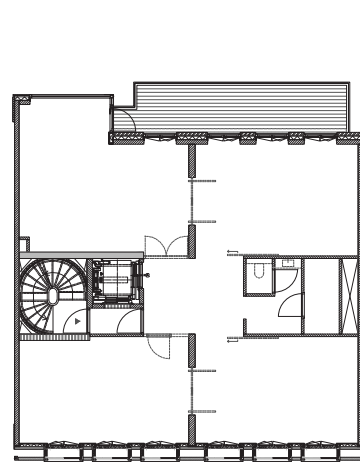
eerste verdieping
