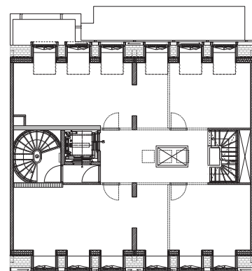
vierde verdieping
