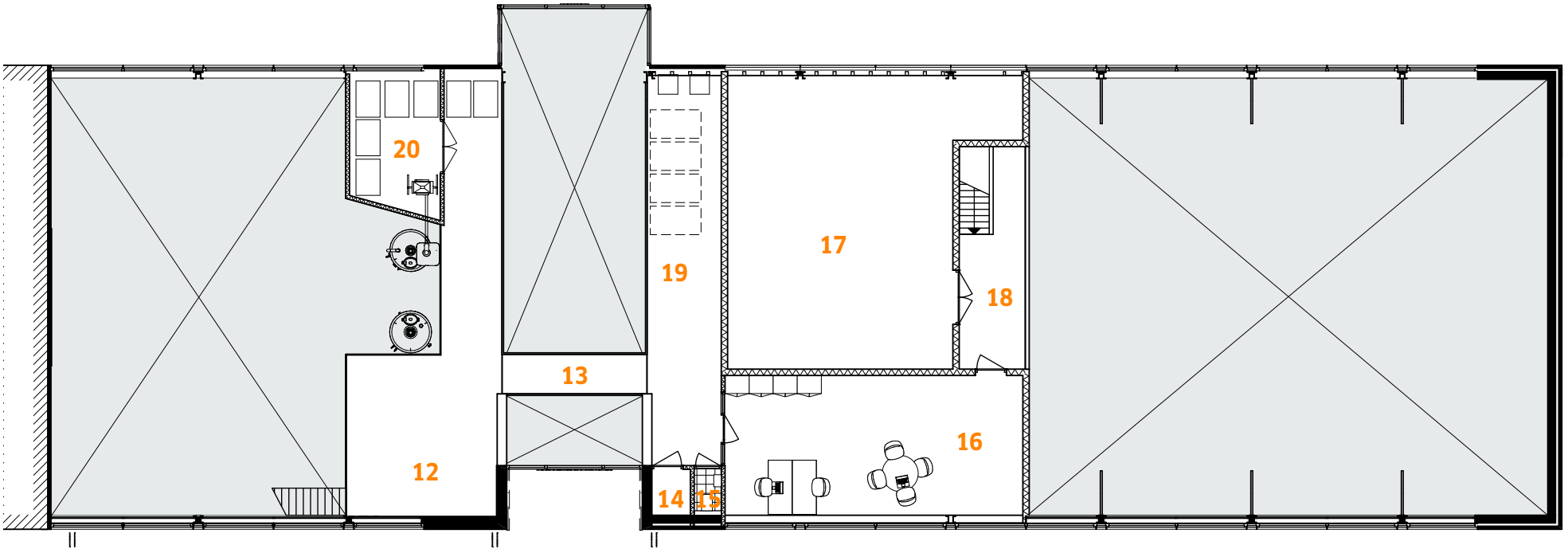
BEGANE GROND
