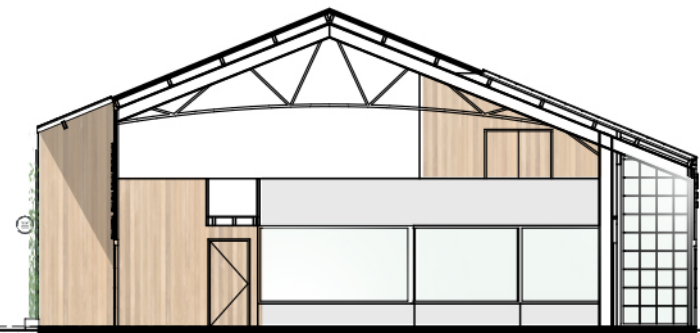
PRINCIPE DOORSNEDE
