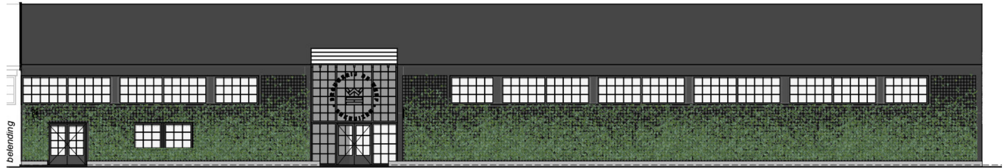
VOORGEVEL - PAKTUINEN
