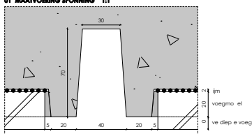
01 MAATVOERING SPONNING 1:1
