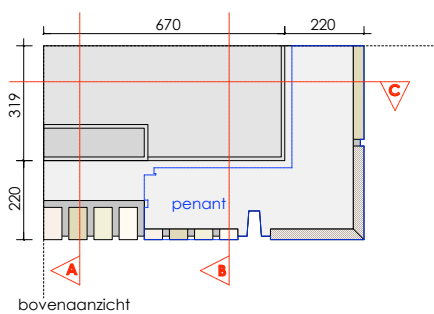
01 MAATVOERING SPONNING 1:1
