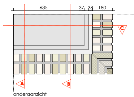
02 PREFAB T.P.V. PUNT 1:1
