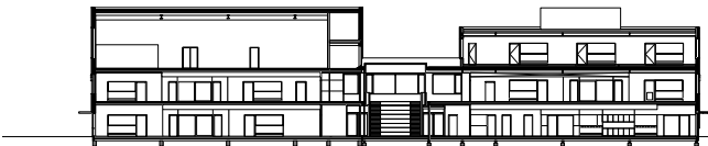
langsdoorsnede
