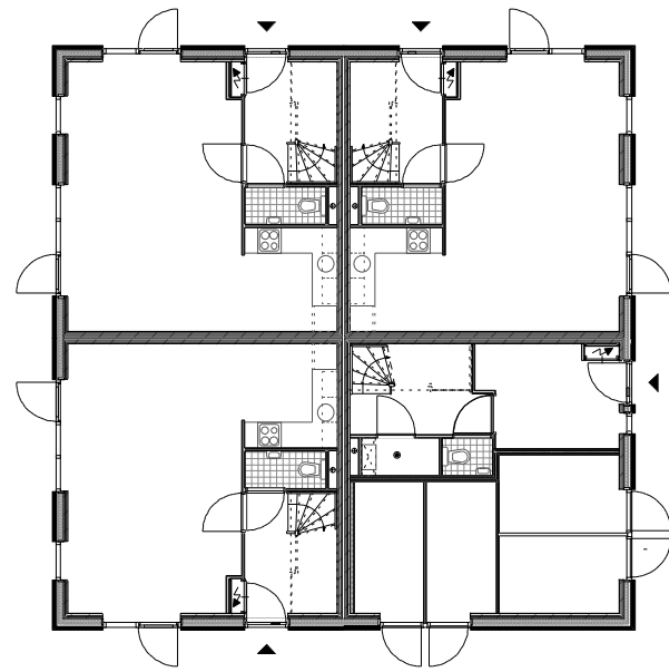
Kwadrantwoning ( 2x 4 woningen )
