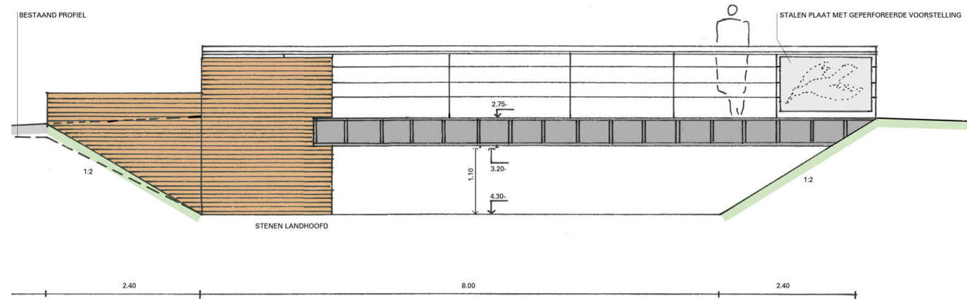
^ ontwerpschets autobridgen < gerealiseerde brug vanaf het Middenpad
