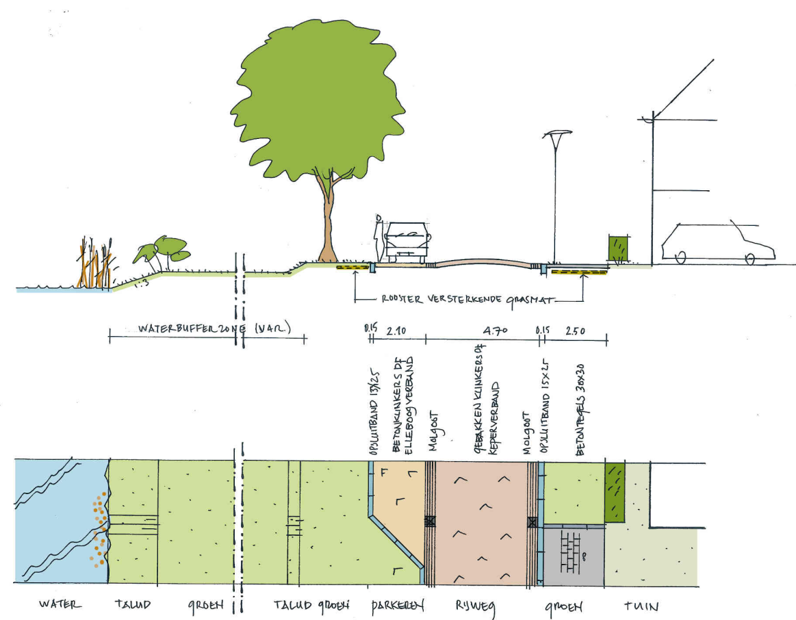
< Dirkjespeerstraat ontwerpschets wegprofielen De Nieuwe Tuinderij >
