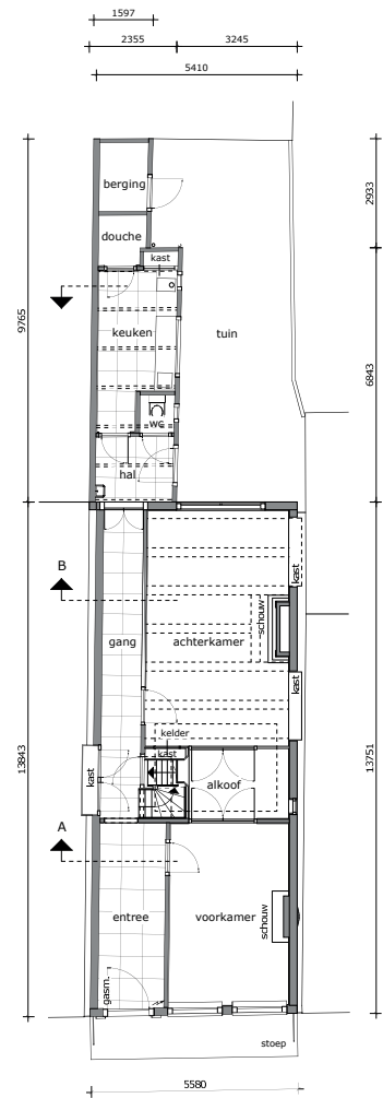
begane grond
