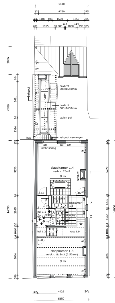
verdieping
