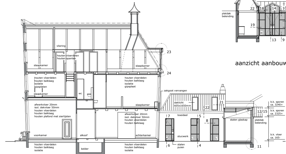
langsdoorsnede
