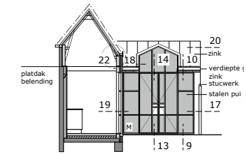
aanzicht aanbouw
