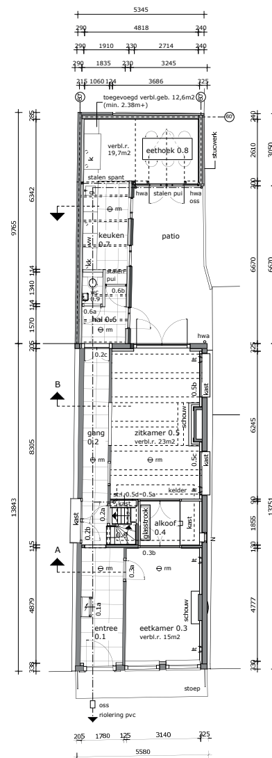
begane grond
