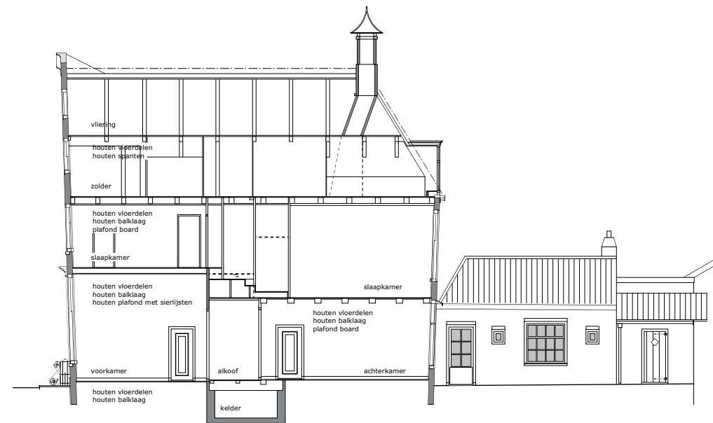
langsdoorsnede
