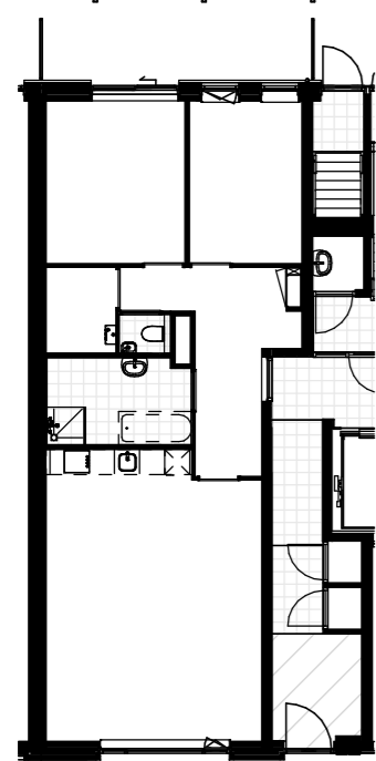
woningtype A1 1 : 200
