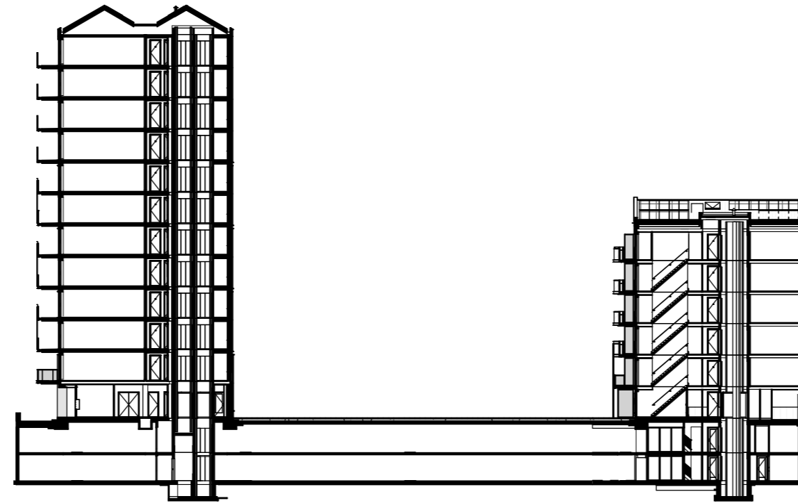
doorsnede 1 : 500
