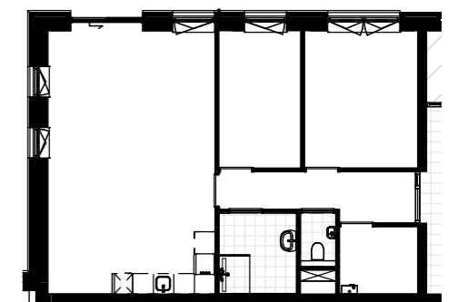
woningtype D5 1 : 200
