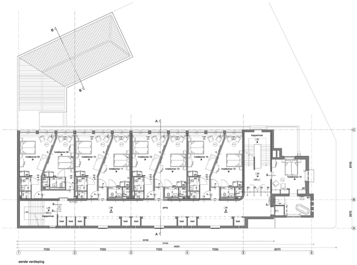
eerste verdieping
